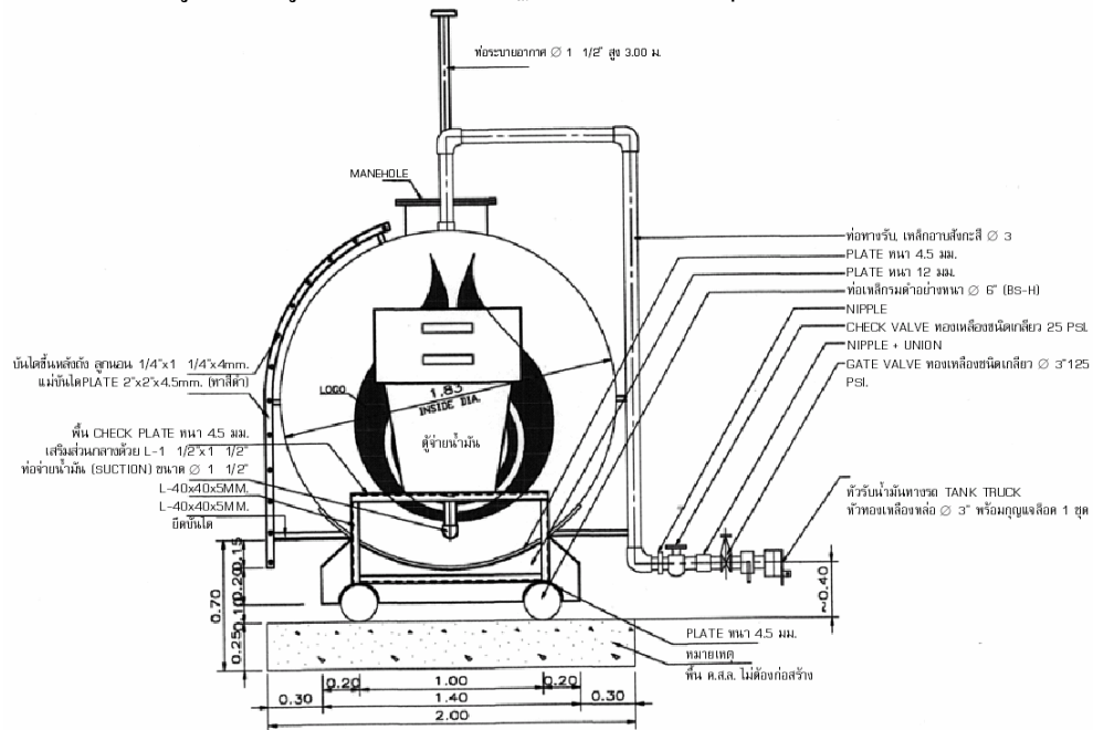
รูปที่ 4-6 รูปด้านหน้าถึงน้ำมันฐานสถิกขนาดบรรจุไม่เกิน 9,600 ลิตร
