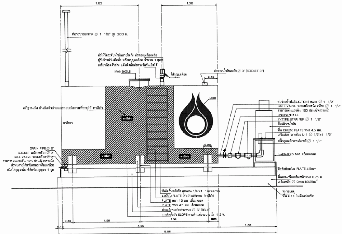
รูปที่ 4-5 รูปด้านข้างถึงน้ำมันฐานสถิกขนาดบรรจุไม่เกิน 9,600 ลิตร
